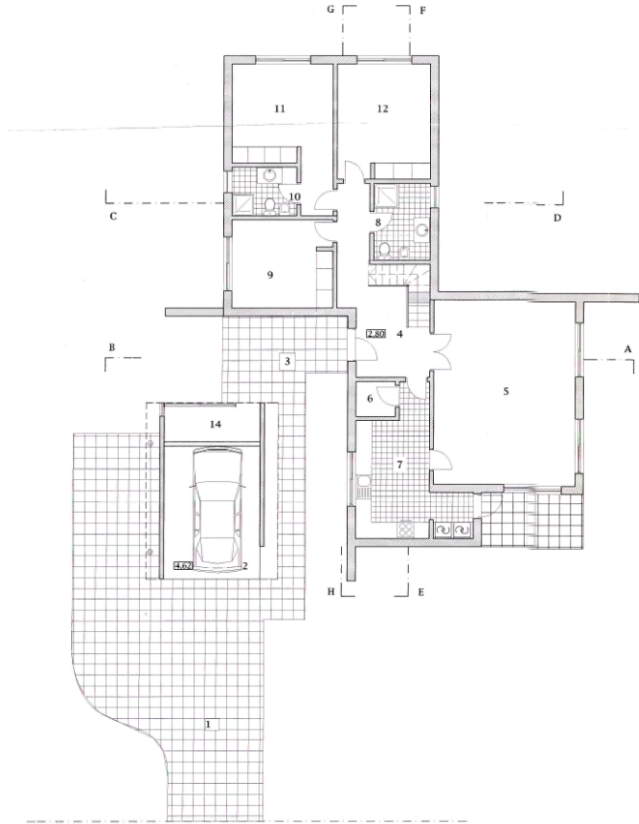
Planta Rés do Chão
