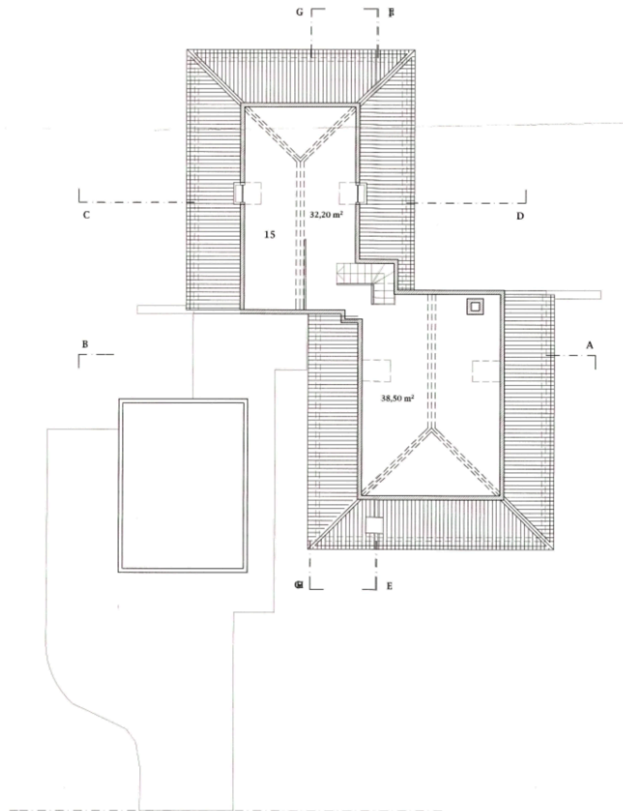
Planta de aproveitamento de cobertura
